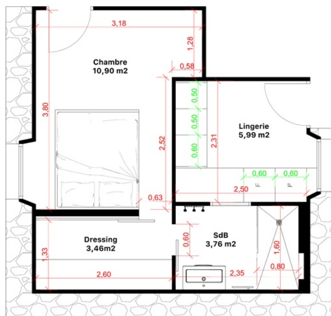
Plan technique côté livré
